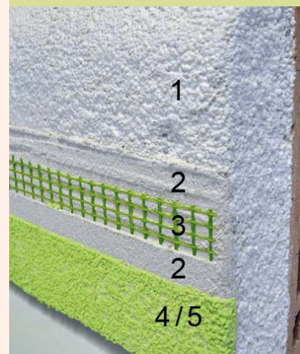
Biotherm Dämmputz
