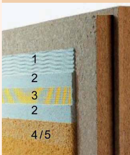
Holzfaserplatten – System
