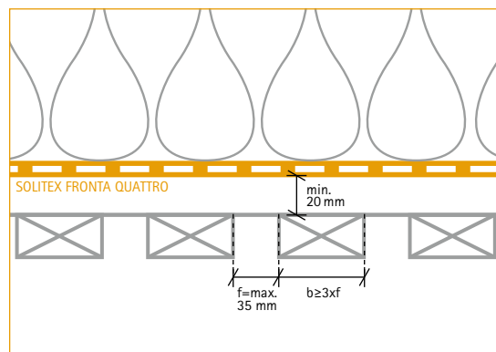
Vertikale Montage
