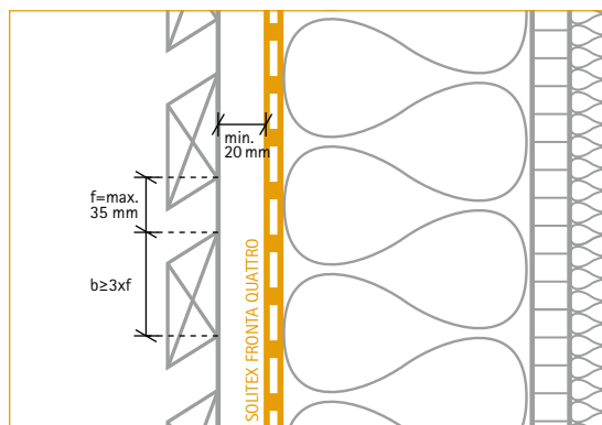
Horizontale Montage
